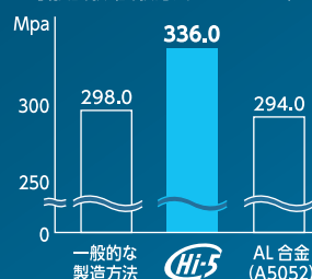
■基本物性 [機械的強度比較] 引張試験 (試験方法 JIS K 7161)
